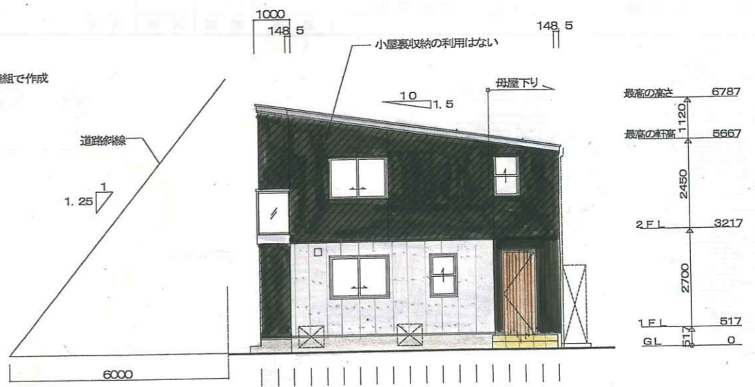
東立面図
