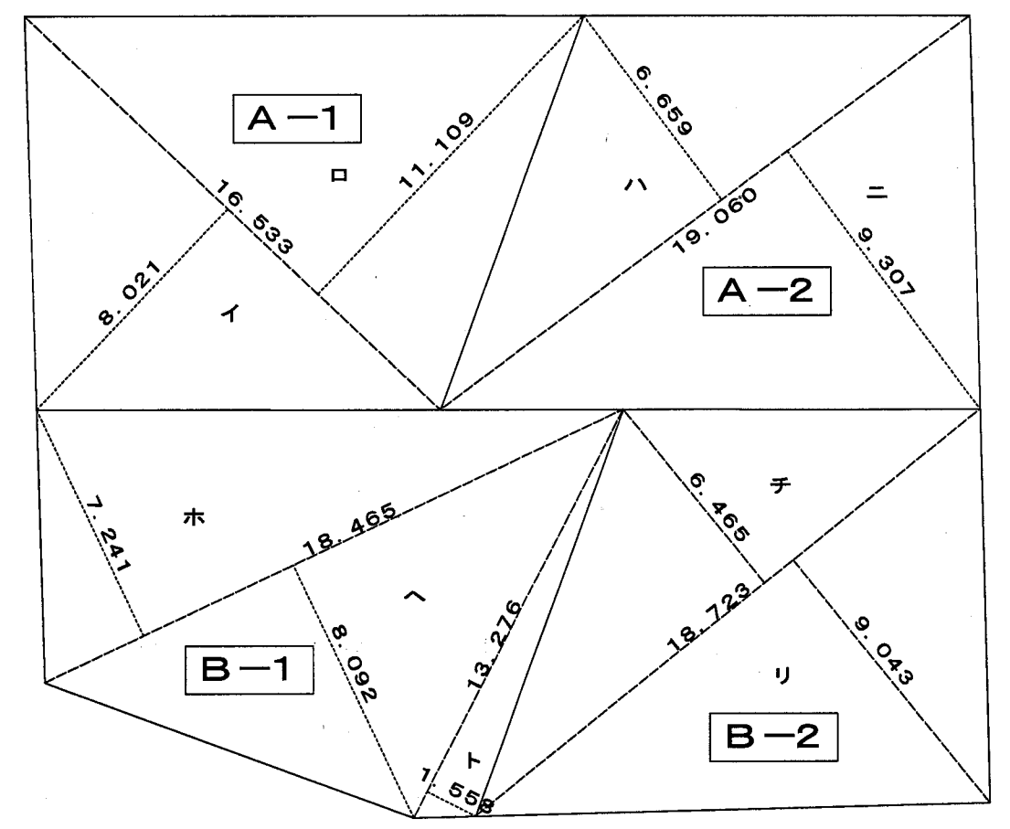
求積図 S=1:200
